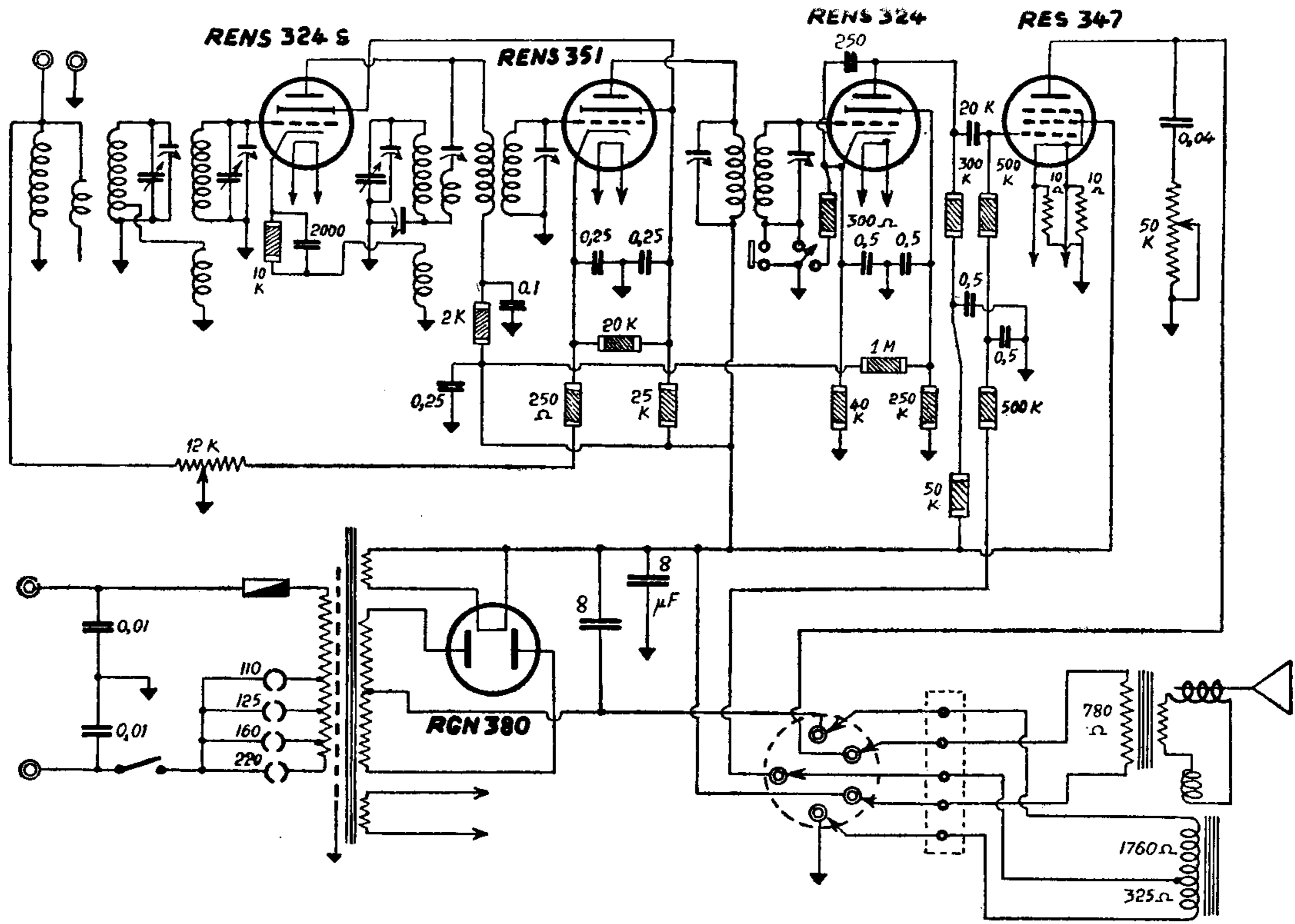
SIEMENS. — Mod. T 540. — Media frequenza: 350 kHz. — Produzione 1932-33.
